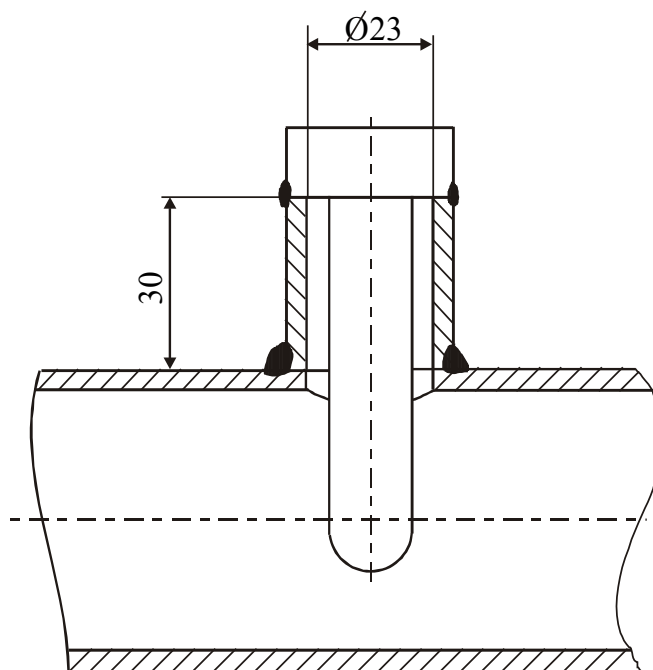
Рисунок 13 - Установка защитной гильзы на трубопроводе при D_u = 50\text{ мм}
