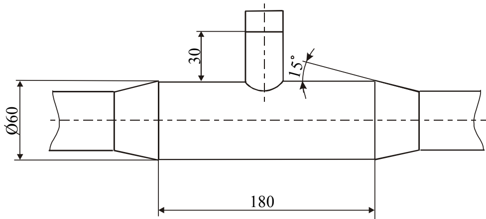
Рисунок 12 - Установка защитной гильзы на трубопроводе при D_u < 50\text{ мм}
