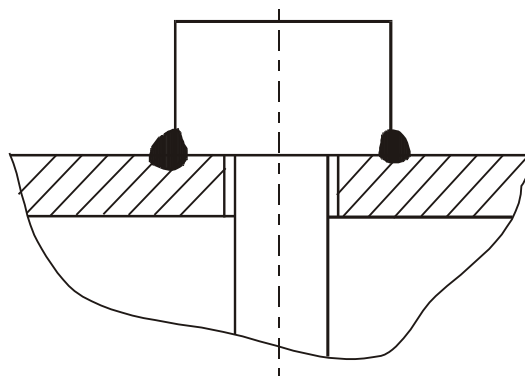
Рисунок 14 - Установка защитной гильзы на трубопроводе при D_u > 50\text{ мм}
