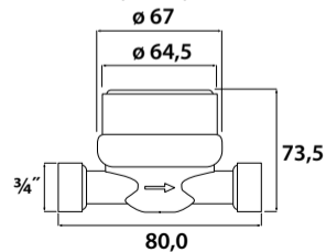
Габаритные и присоединительные размеры
